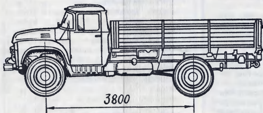
Бортовой автомобиль. Базовая модель ЗИЛ—130-76.
