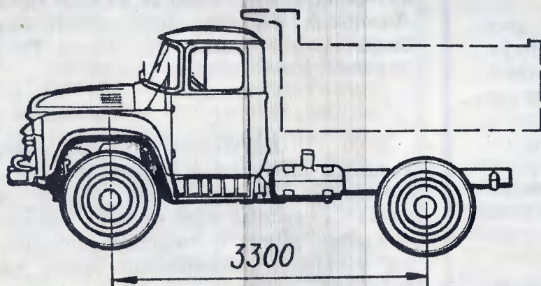
Шасси строительного самосвала ЗИЛ—130Д1 (и 130Д2).
