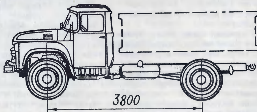
Шасси сельскохозяйственного самосвала ЗИЛ—130Б2.
