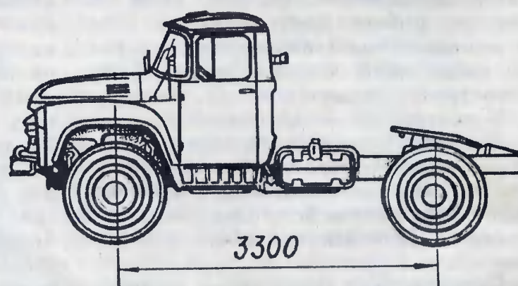
Седельный тягач ЗИЛ—130В1.
